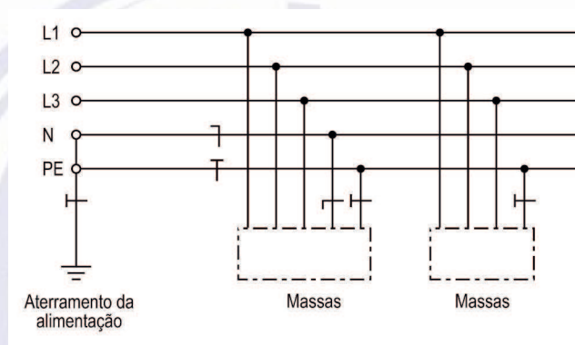
Figura 1 — Esquema TN-S
