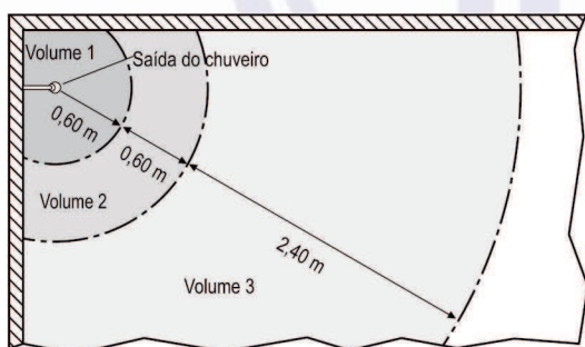
Figura 17 — Dimensões dos volumes — Chuveiro ou ducha, com piso-boxe
