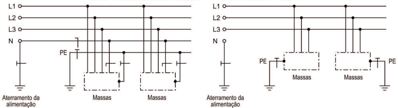
Figura 4 — Esquema TT
