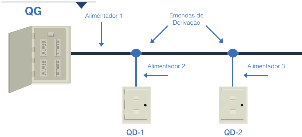
Figura 37: Circuitos com mesma seção nominal
