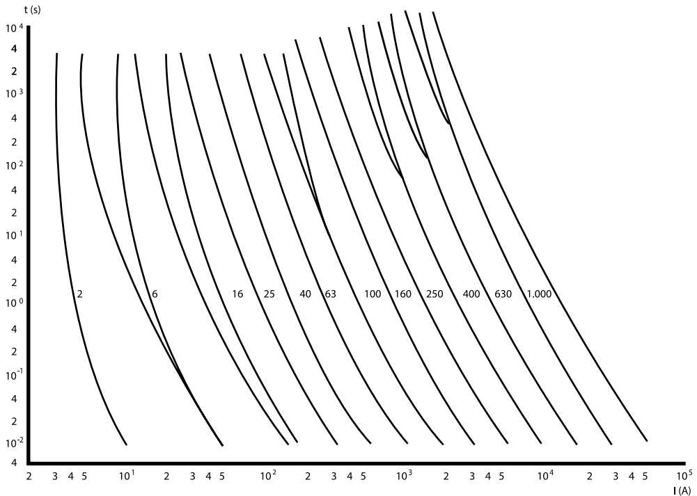
Figura B1: Fusíveis gG – NBR IEC 60269-2 e 3
