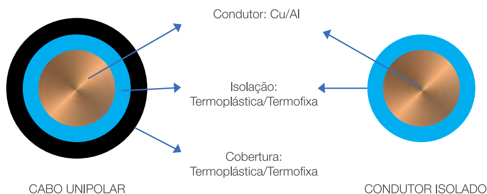
Figura 8: Construção típica de condutores de baixa tensão
