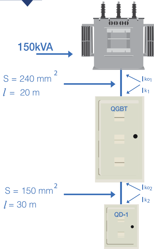
Figura 47: Circuito para cálculo simplificado da corrente de curto-circuito presumida
