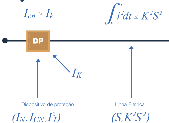
Figura 40: Condição geral de proteção contra curto-circuito
