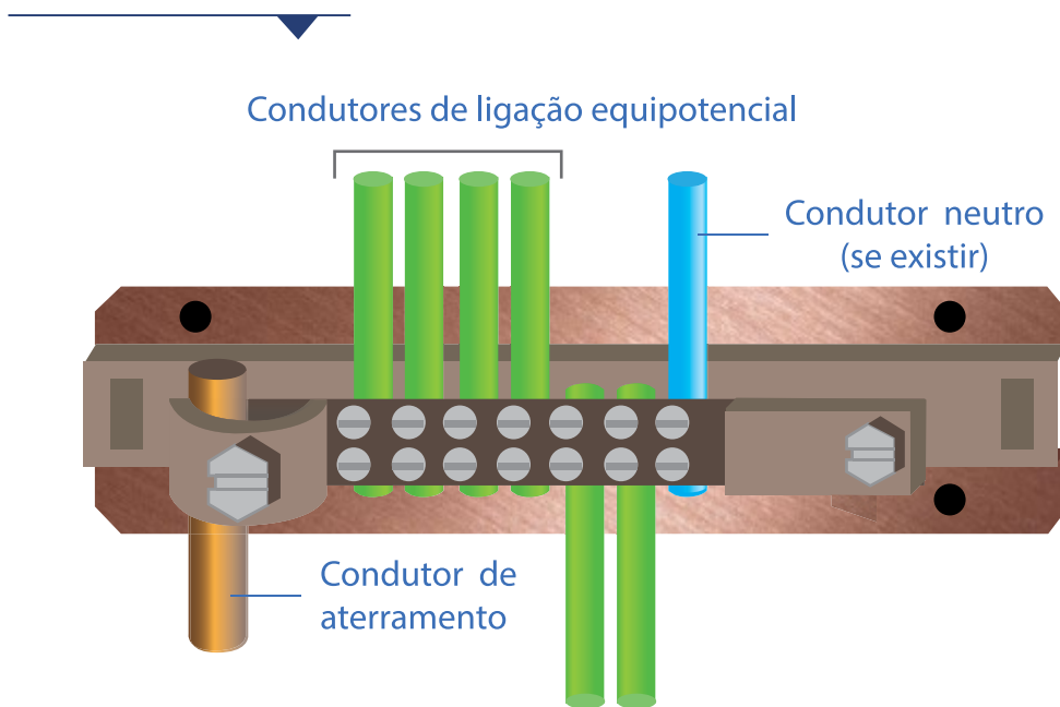
Figura 54: As dimensões físicas de um BEP na forma de barra dependem de cada projeto
