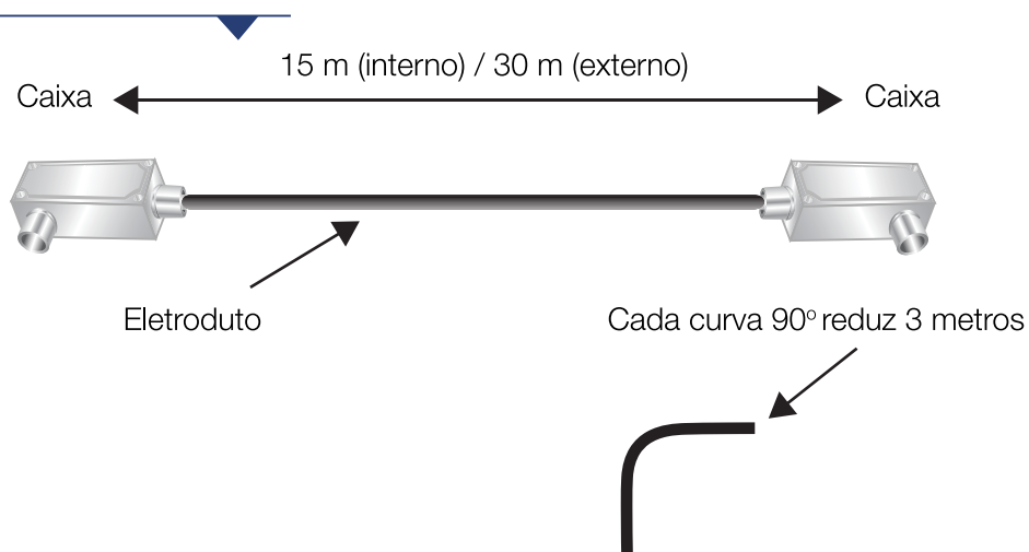
Figura 22: Distâncias para instalação de caixas em eletrodutos
