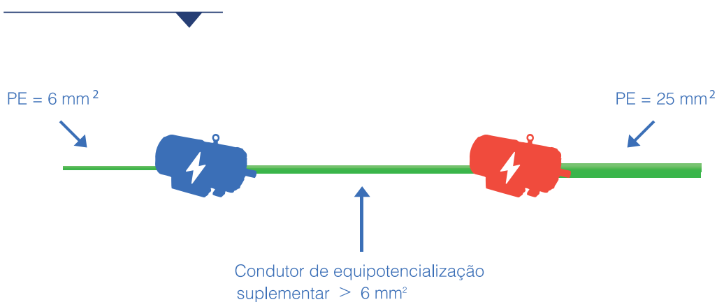
Figura 52 - Exemplo de dimensionamento de condutor de equipotencialização entre duas massas
