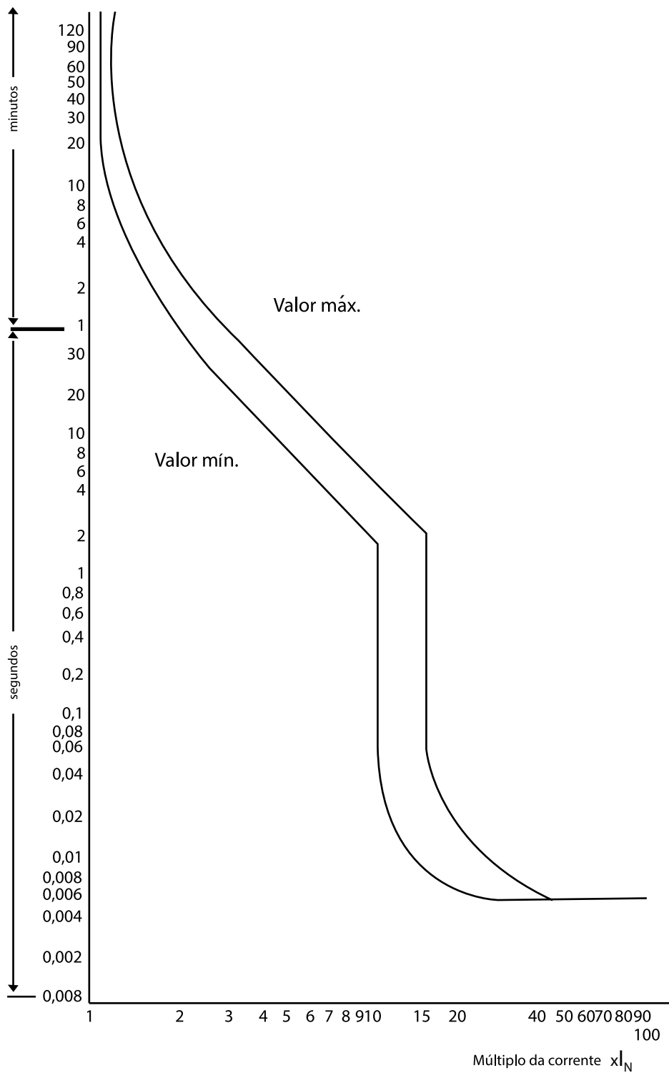
Figura B3: Disjuntores NBR IEC 60947-2 e RTQ 243
