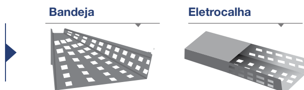
Figura 4: A diferença entre eletrocalha e bandeja é a presença ou não da tampa
