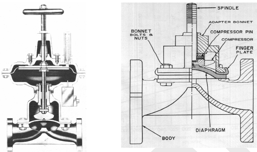
Válvula Tipo Diafragma
