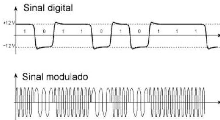
Figura 4 - Modulação de um sinal digital.
