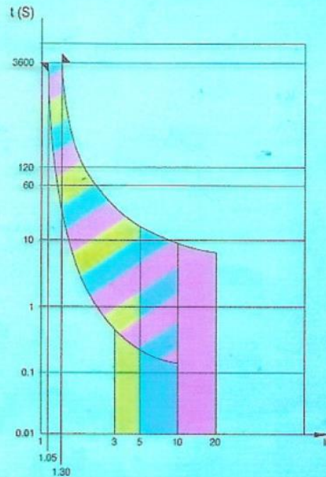
IEC 947-2: Curva de Disparo
