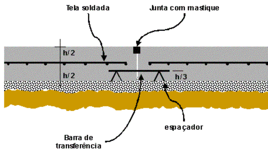
Figura 21. Piso de concreto armado.
