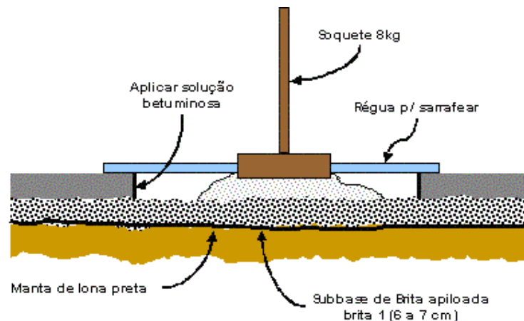
Figura 3. Contrapiso sobre o solo.
