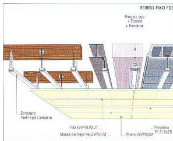
Figura 2. Forro de gesso acartonado fixo por perfis metálicos.
