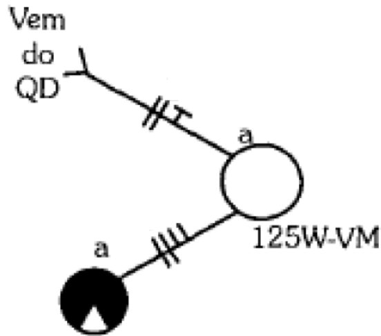
Figura 150 – Esquema unifilar de alimentação da lâmpada de vapor de mercúrio.
