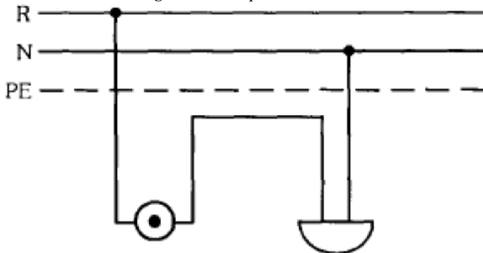
Figura 159 – Esquema multifilar.
