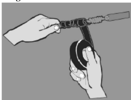
Figura 93 – Isolando a emenda.
