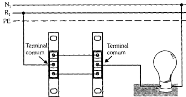
Figura 141 – Esquema multifilar.
