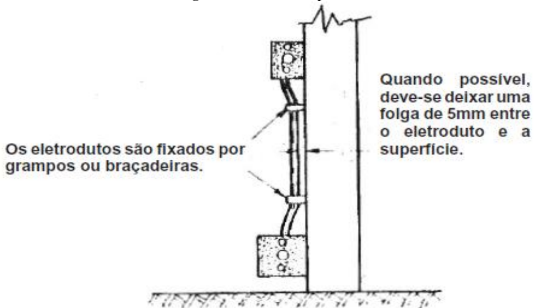
Figura 112 - Rede exposta.
