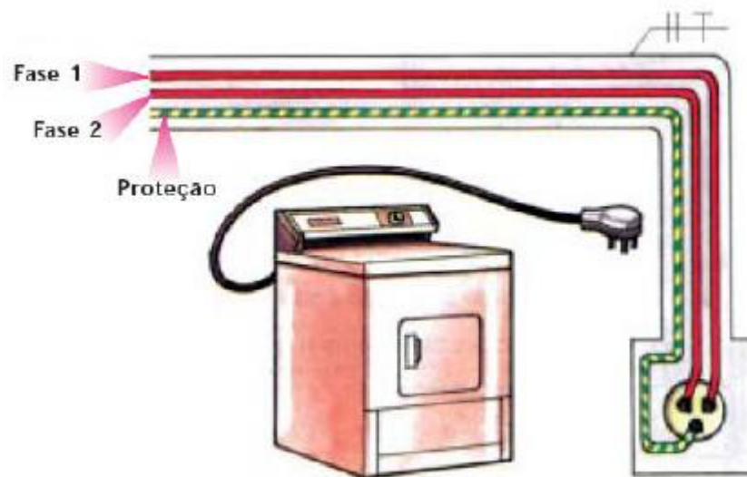
Figura 123 – Tomada bifásica.
