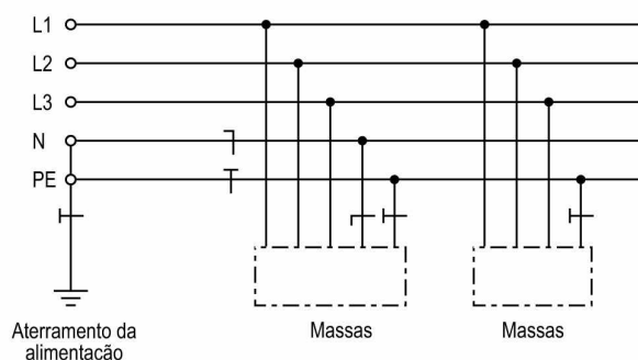
Figura 1 — Esquema TN-S
