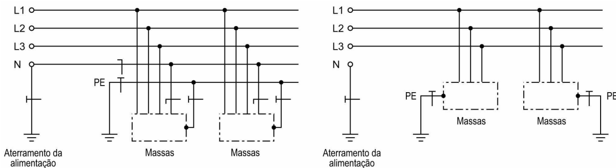
Figura 4 — Esquema TT
