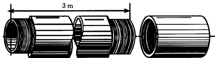
Figura - Detalhe do Eletroduto e Luva de PVC Rígido Roscável
