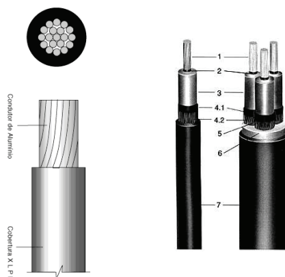
Figura 5 – Tipos de fios e cabos condutores.
