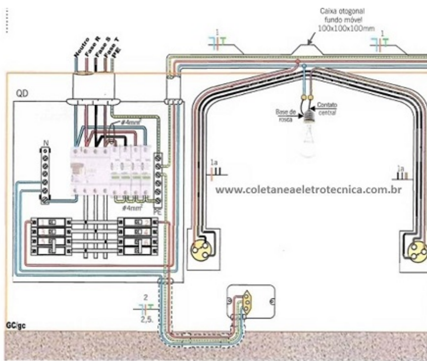
Quadro de distribuição com pontos de utilização.
