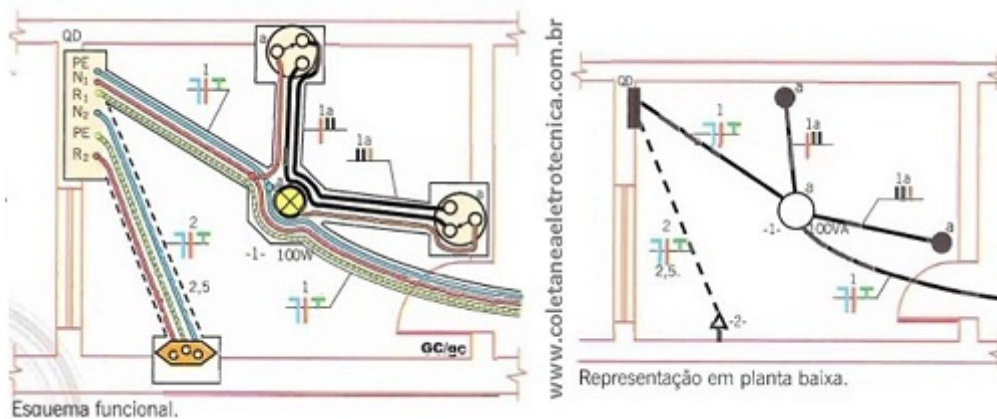
Esquema funcional.
