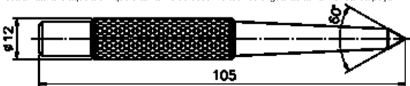
Punção com dimensões em milímetros - ESC.: 1:1
